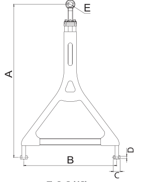
Tip 3 - Çeki Oku Type 3 - Drawbar Eye
